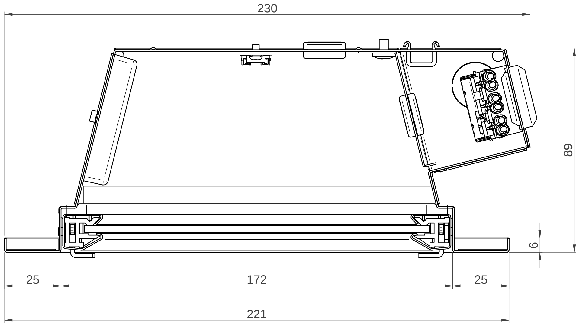
SEZIONE TRASVERSALE
